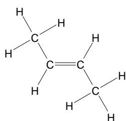
E-but-2-ene
